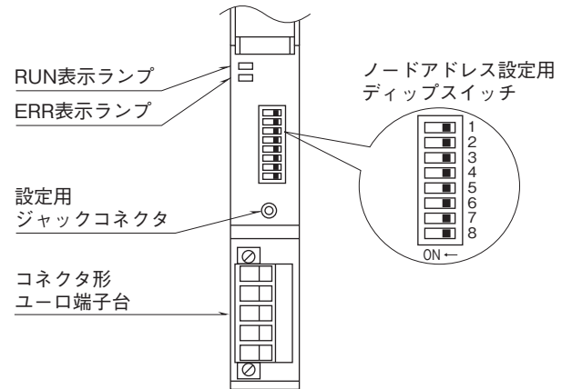
■前面図
