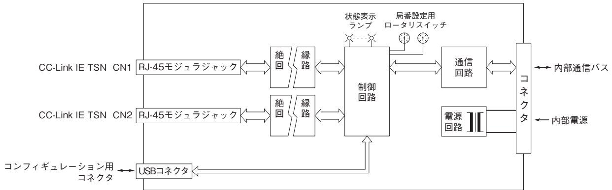
CC-Link IE TSN 通信用 RJ-45 モジュラジャックのCN1とCN2は、配線の接続順序に制約はありません。
