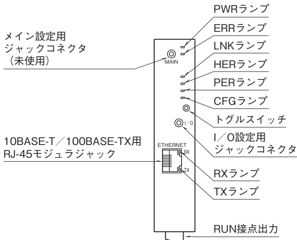
■前面図
