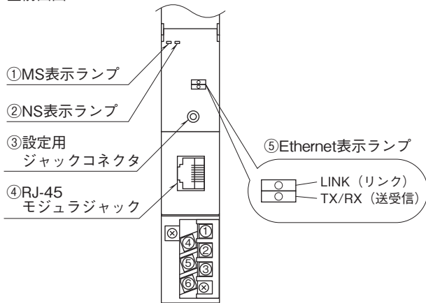
■前面図
