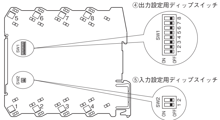
■側面図
