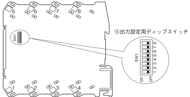
■側面図
