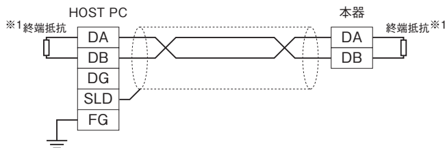
■HOST PCとの配線
