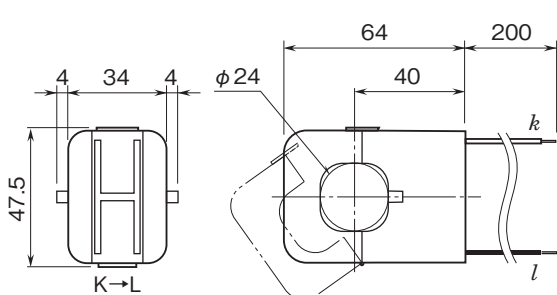
■クランプ式センサ:CLSA-30
