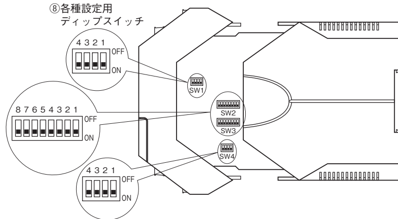
■側面図
