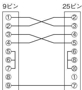
■配線図
