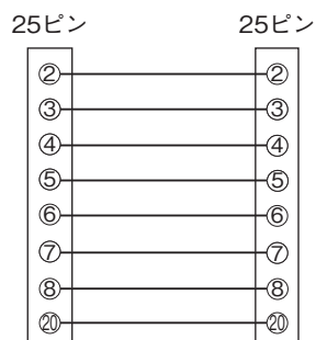
■配線図
