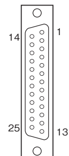
■コネクタピン配列
