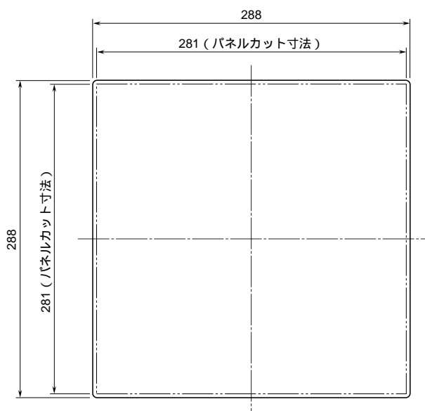
前面図
