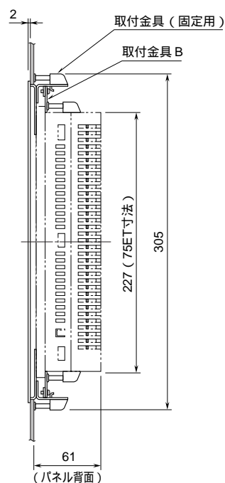
側面図
