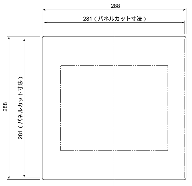
前面図
