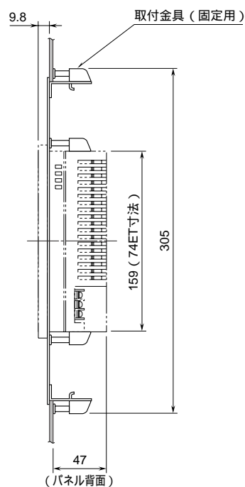
側面図
