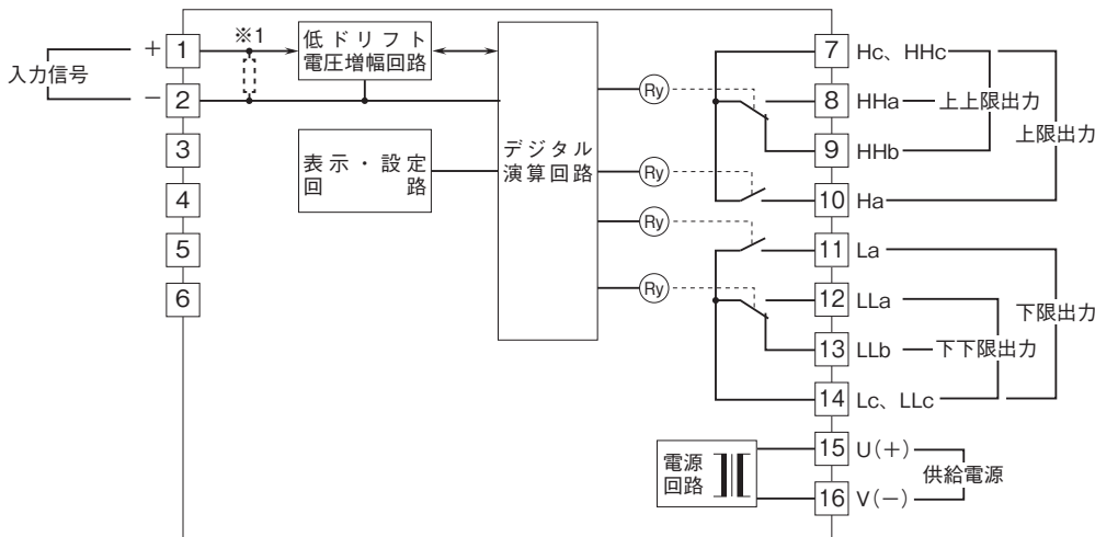
■48NAV-4 (4点警報/4接点出力)
