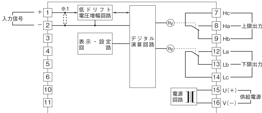
■48NAV-2 (2点警報/2接点出力)
