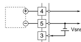
電圧パルス入力
