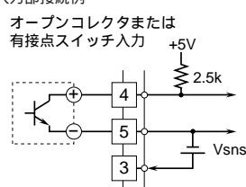
入力部接続例
