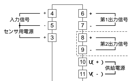
入力部接続例
