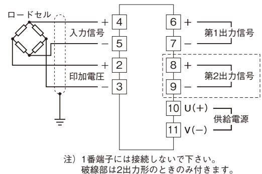
端子接続図
