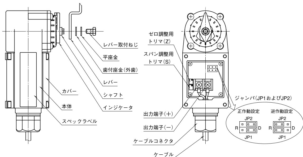
図1 各部の名称
