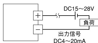
図5 端子接続図
