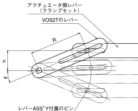
図3 レバー回転角とストロークの関係
