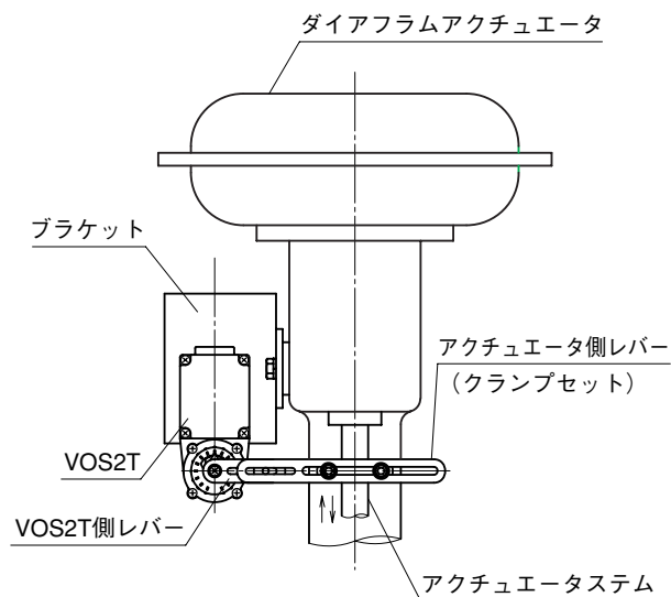
図4 VOS2T取付例
