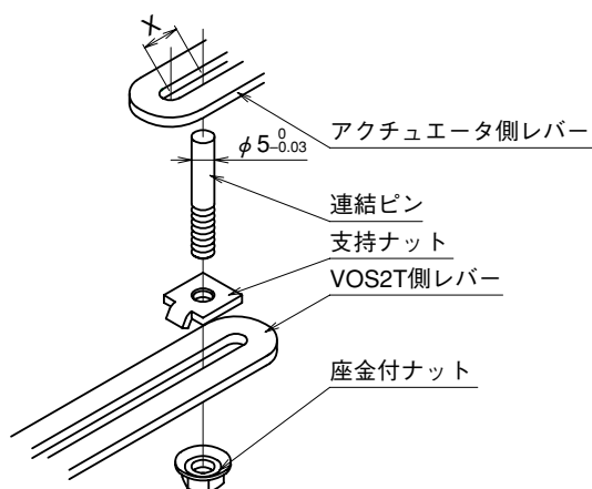
図2 連結ピン取付
