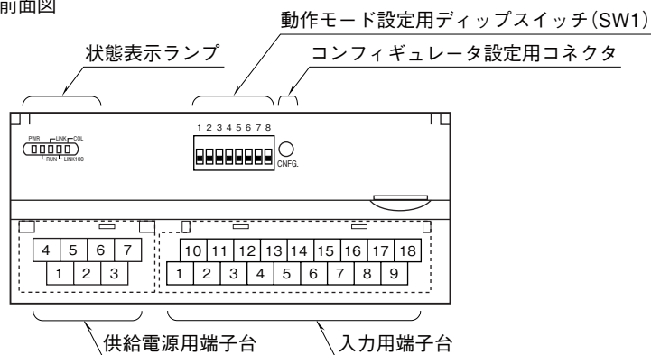
■前面図
