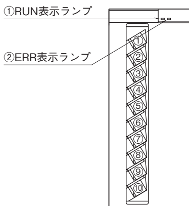
■前面図
