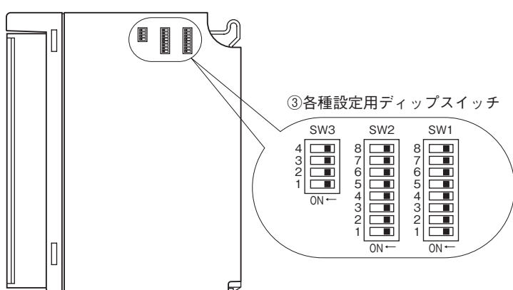
■側面図
