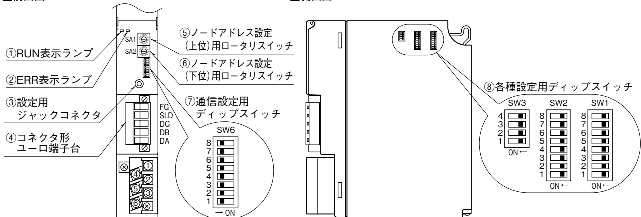
■前面図
