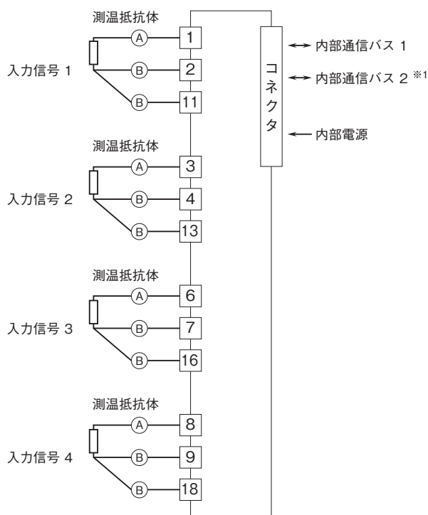
端子接続図
