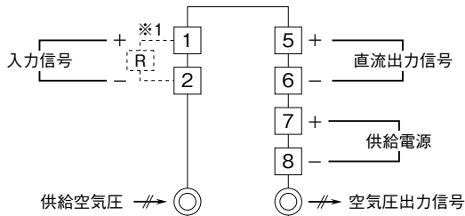
端子接続図
