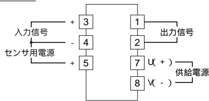
端子接続図
