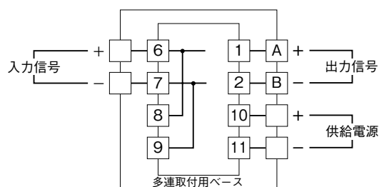
端子接続図
