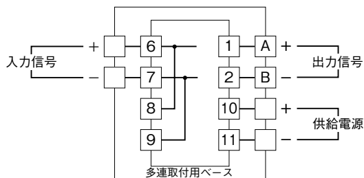
端子接続図
