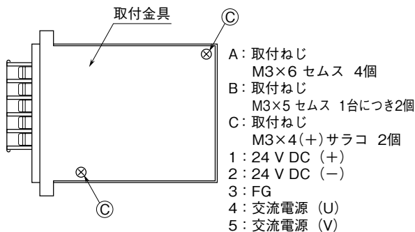
●HDC4-□-R 側面図
