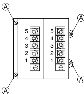
●前面図
