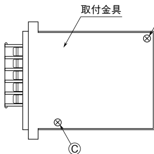
●HDC4-□-R 側面図
