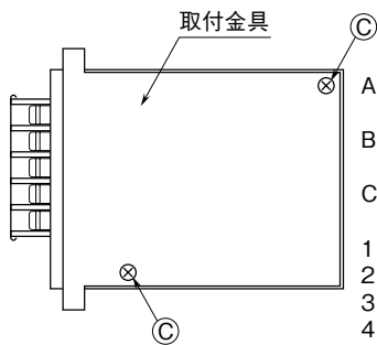
●HDC4-□-R 側面図
