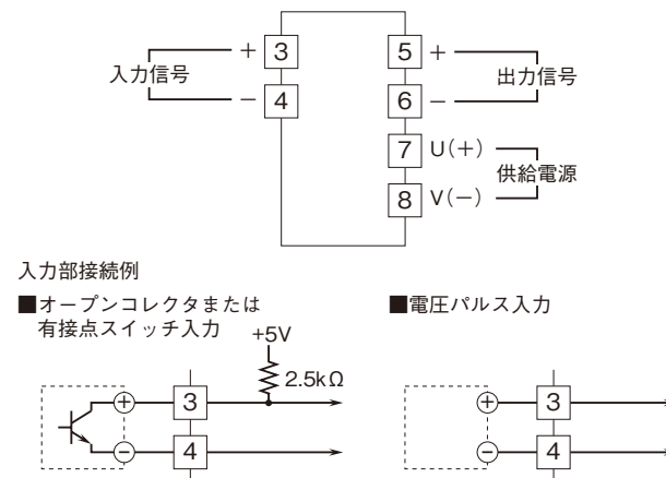
端子接続図
