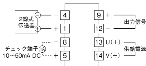
端子接続図
