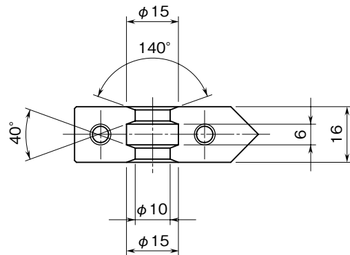
図9 インジケータ詳細図
