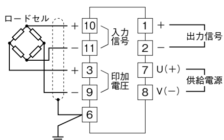
端子接続図
