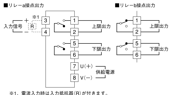
端子接続図
