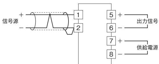
端子接続図
