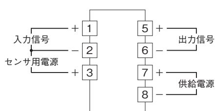
端子接続図
