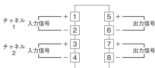
端子接続図
