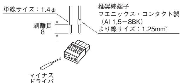
■コネクタ形ユーロ端子台の接続
