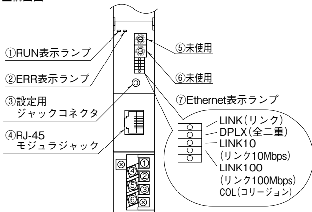
■前面図
