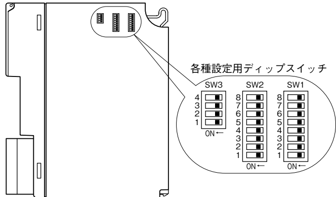
■側面図
