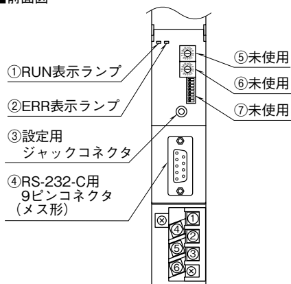
■前面図
