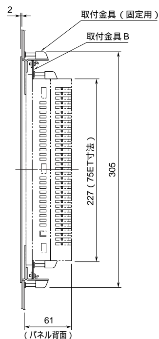
側面図
