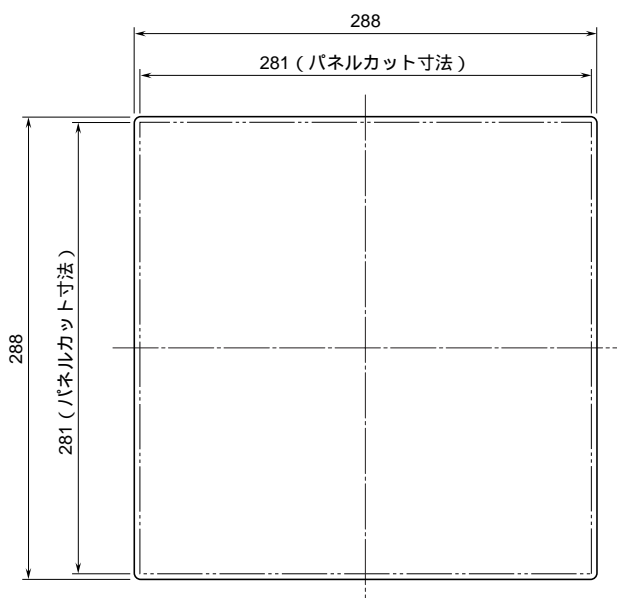
前面図
