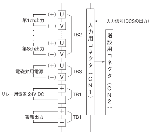
端子接続図
