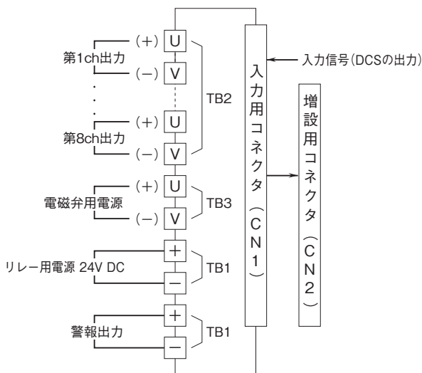
端子接続図
