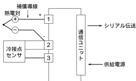
端子接続図
