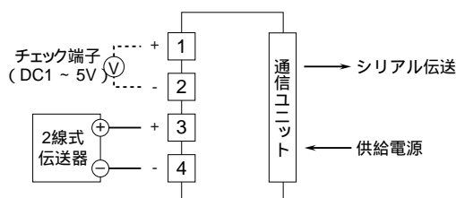
端子接続図
