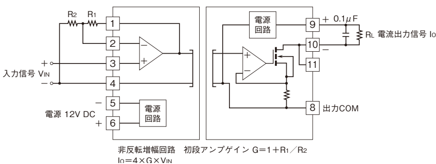
■非反転増幅回路：非反転増幅回路例
