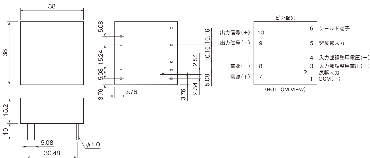
外形寸法図 (単位: mm) ・端子番号図
