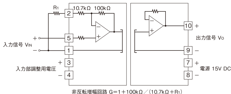
非反転増幅回路 G=1+100\text{ k}\Omega / (10.7\text{ k}\Omega + R_1)
