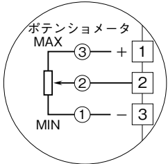
図A フィールド用端子接続図
