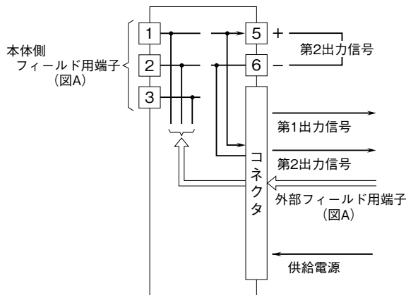
図A フィールド用端子接続図
