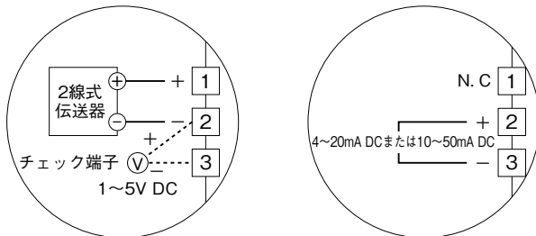
図A フィールド用端子接続図
