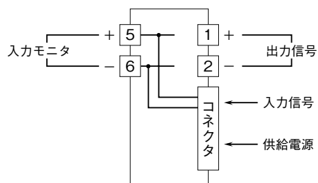
端子接続図
