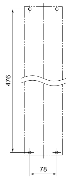
取付寸法図（単位：mm）
